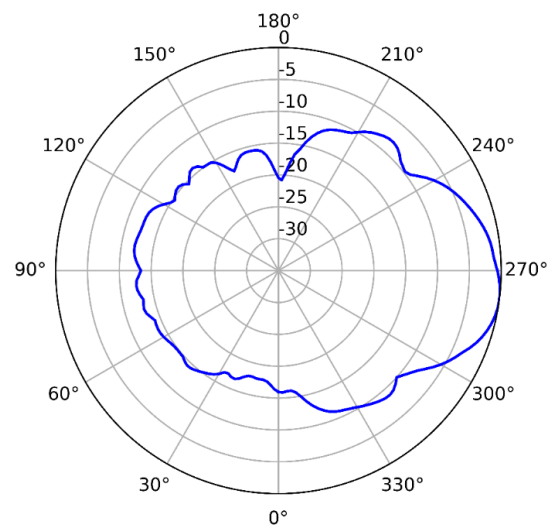
2.4GHz (Vertical)
